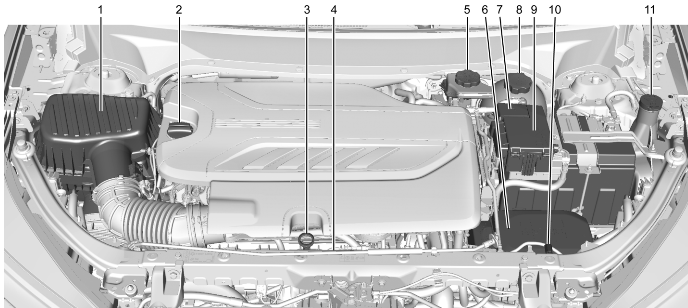
Двигатель LХН объемом 2.0 л
